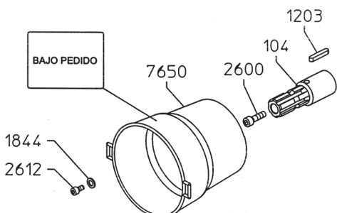
MODELO CARDÁN LADO TRASERO
