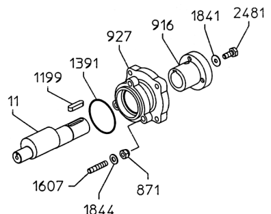
VARIANTES RO 106 VA RESPECTO A RO 106 1C
